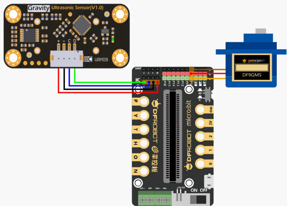
图 4.4.1 连线示意图
