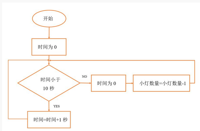
图 2.4.8 彩灯倒计时部分逻辑图
