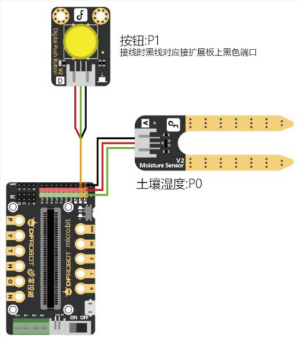
图 3.2.4 连线示意图
