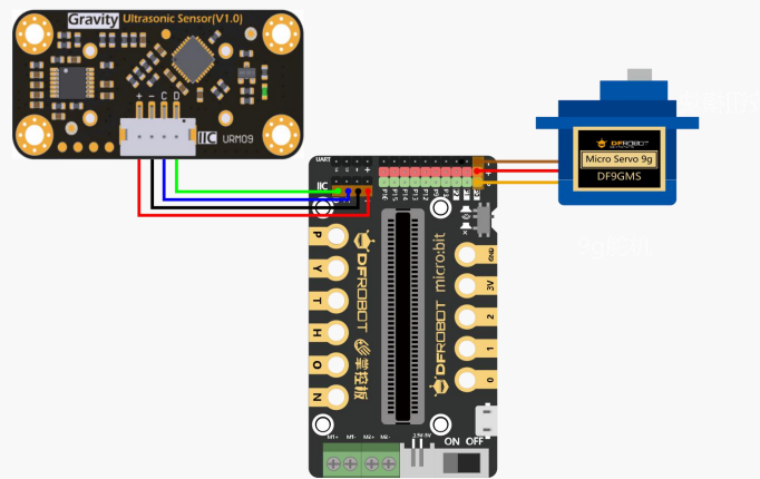
图 3.3.3 连线示意图
