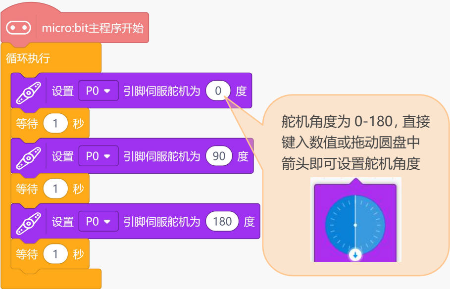
图 3.3.2 舵机转动
