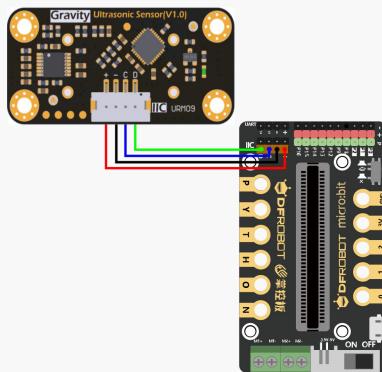
图 3.1.1 接线示意图
