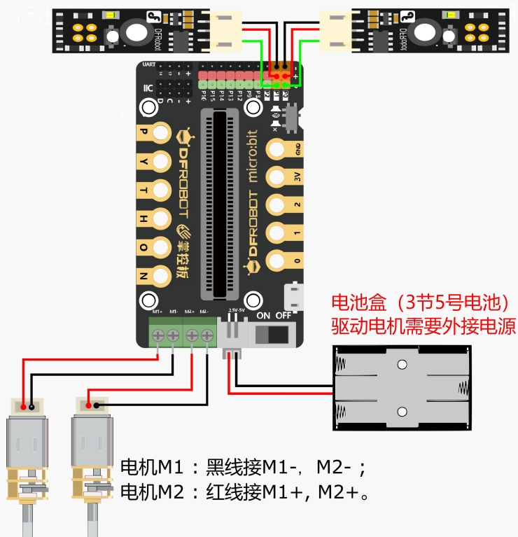
图 4.3.2 连线示意图
