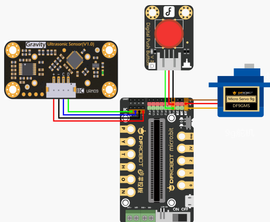
图 3.3.5 连线示意图
