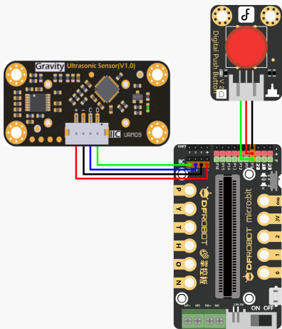
图 3.1.5 连线示意图
