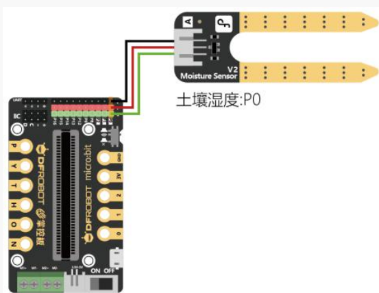
图 3.2.1 连线示意图
