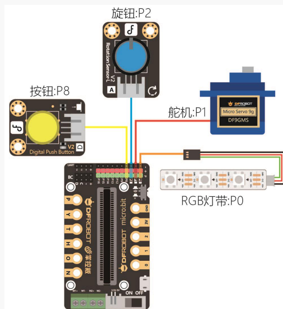
图 3.4.3 连线示意图
