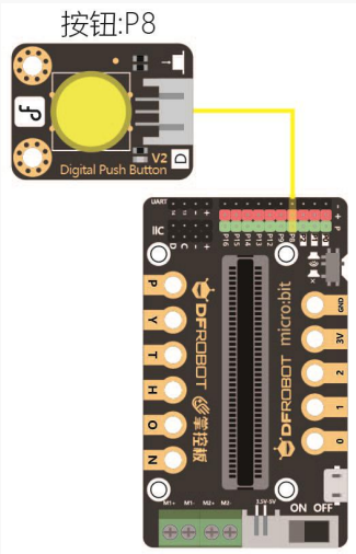
图 3.4.1 连线示意图
