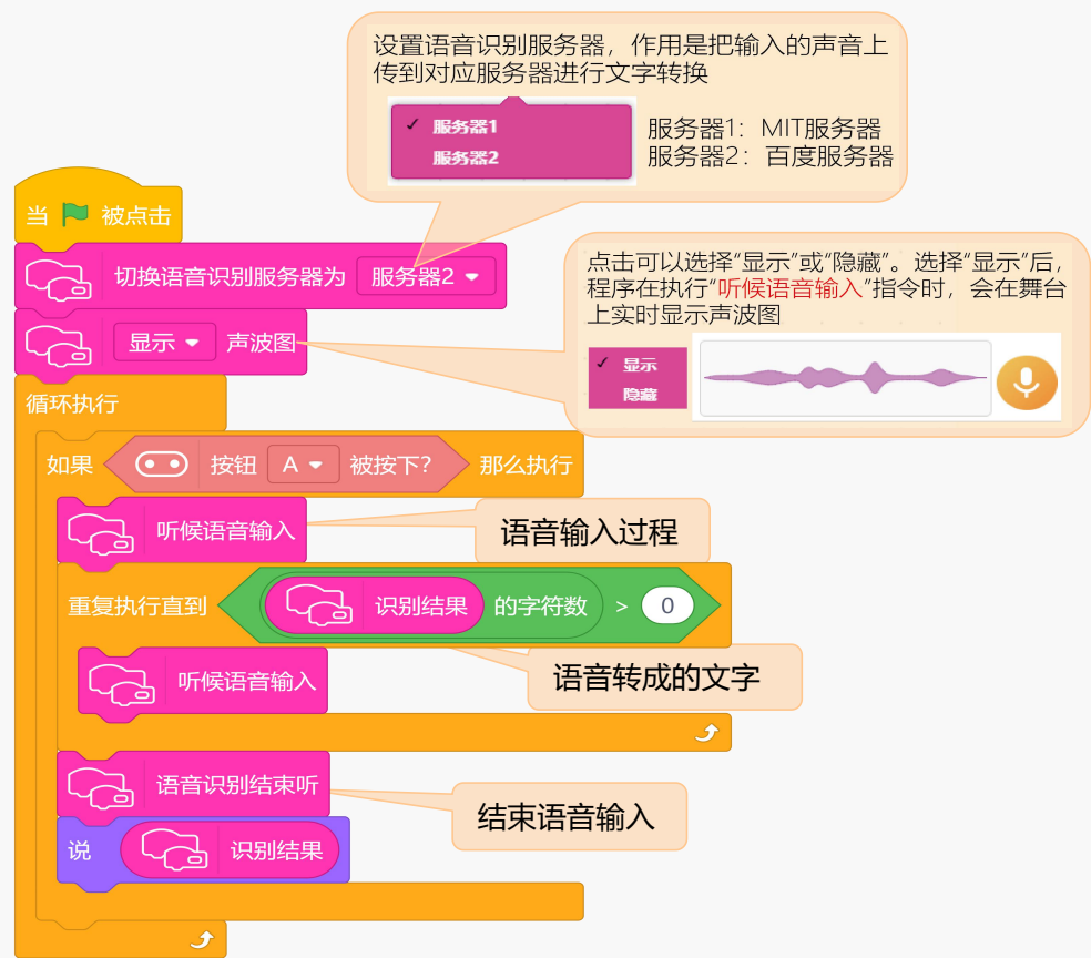
图 4.2.3 执行程序说明
