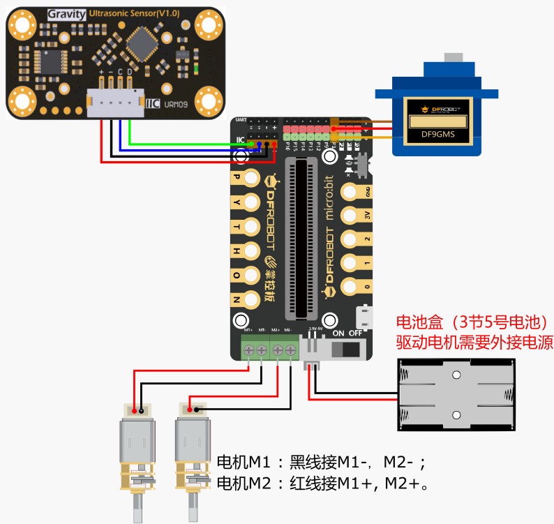
图 4.4.3 连线示意图
