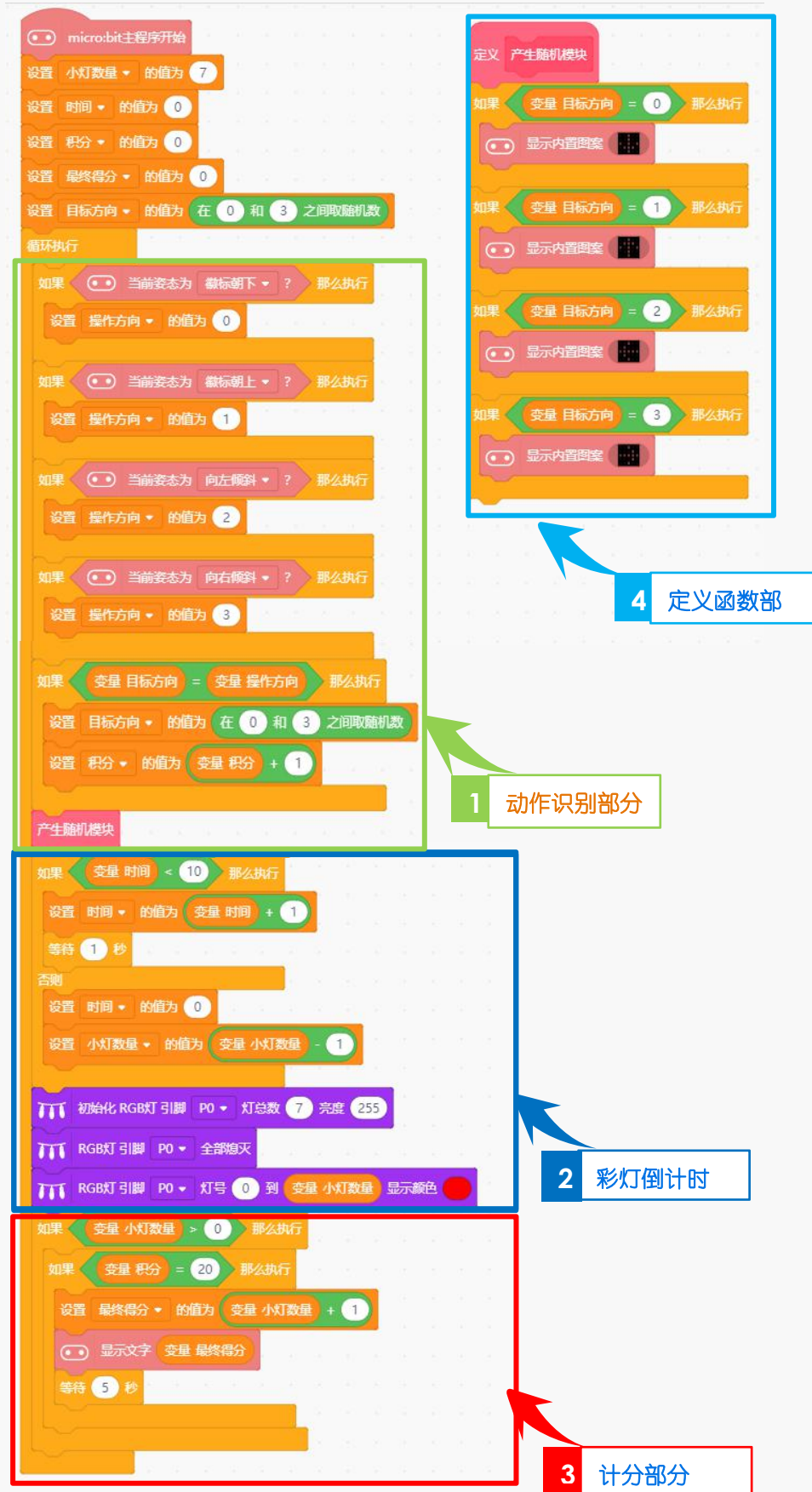
图 2.4.14 完整执行程序
