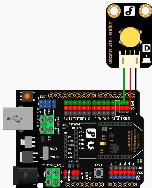
图 2.3.1 硬件连接图
