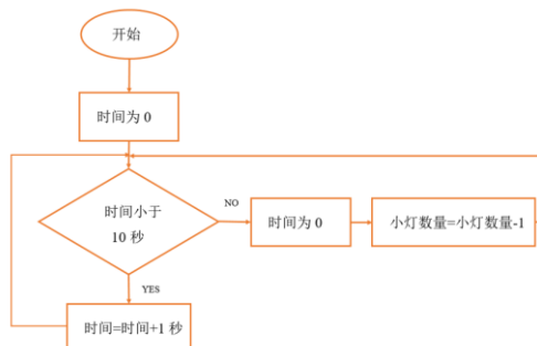
图 4.4.8 彩灯倒计时部分逻辑图
