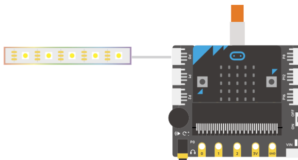
图 4.4.1 连线示意图
