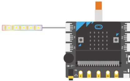
图 3.4.1 接线示意图
