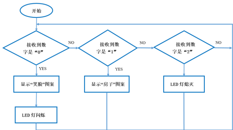
图 4.3.5 接收端逻辑图
