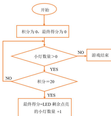
图 4.4.12 计分部分逻辑图
