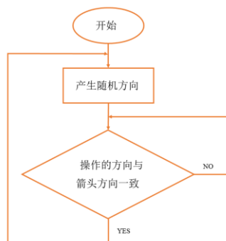
图 4.4.2 动作识别部分逻辑图
