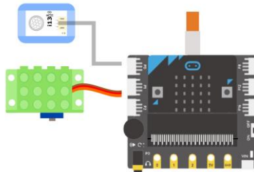
图 3.2.9 连线示意图
