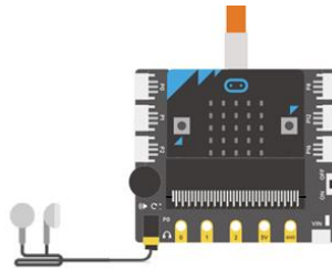
图 3.3.1 接线示意图
