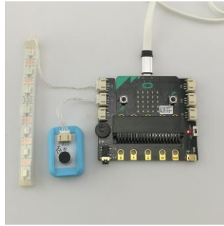
图 3.4.14 连线示意图
