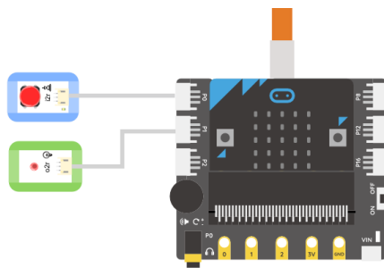
图 2.3.1 接线示意图
