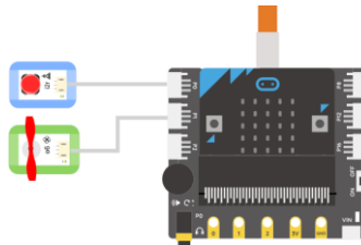
图 2.4.1 接线示意图
