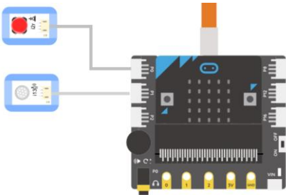
图 4.3.1 发射端连接示意图
