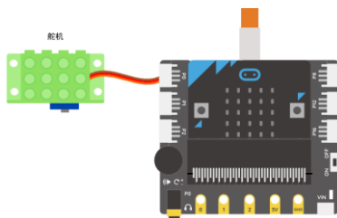
图 4.1.3 连接示意图
