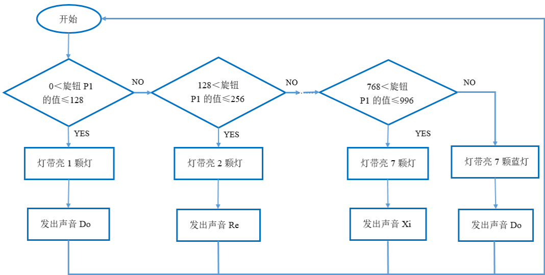
图 4.2.2 逻辑图
