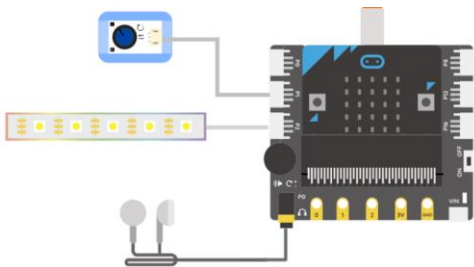
图 4.2.1 连线示意图
