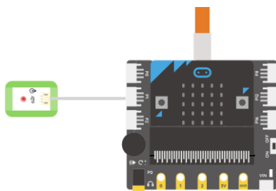
图 2.2.3 连接 LED 灯
