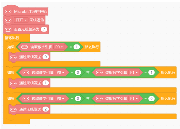
图 4.3.4 发射端执行程序
