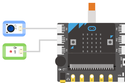
图 2.3.7 连线示意图
