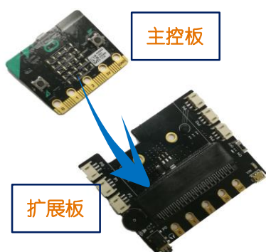
图 2.2.1 连接方法
