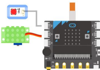
图 3.2.1 接线示意图
