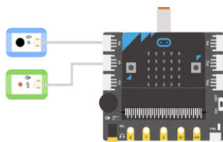
图 3.1.1 接线示意图
