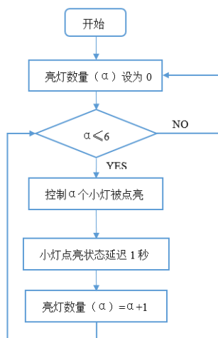
图 3.4.10 逻辑图
