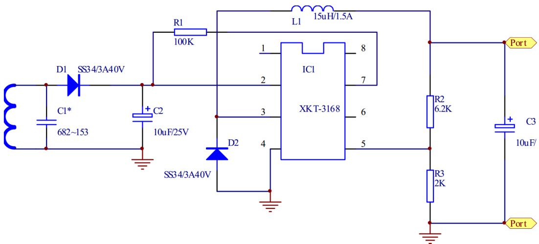
接收电路原理图
