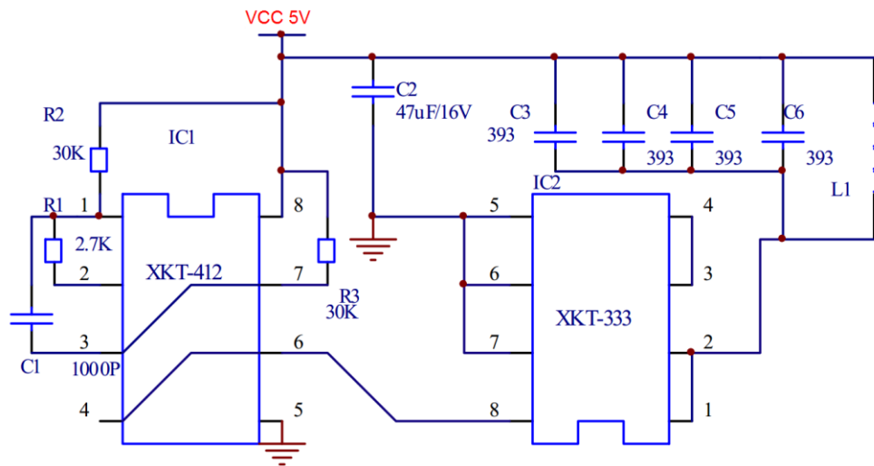
接收电路原理图
