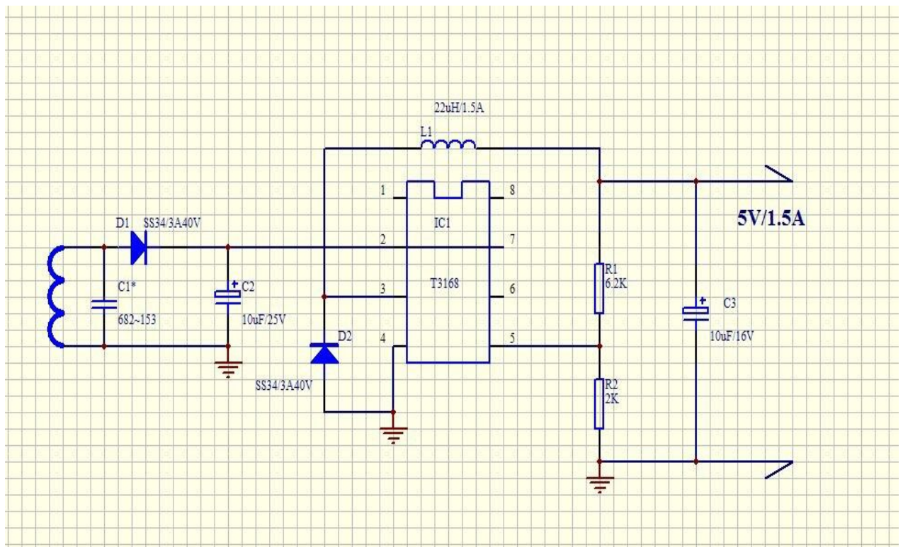
模块接收原理图
