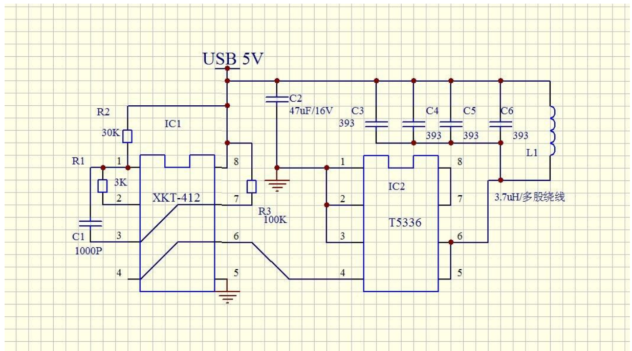
模块发射原理图
