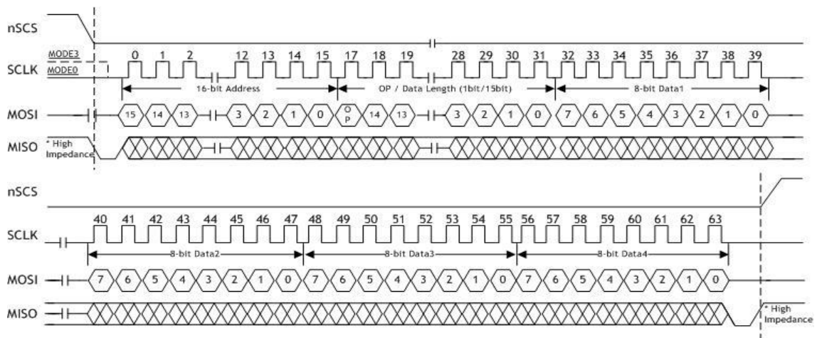
图 21 读时序
