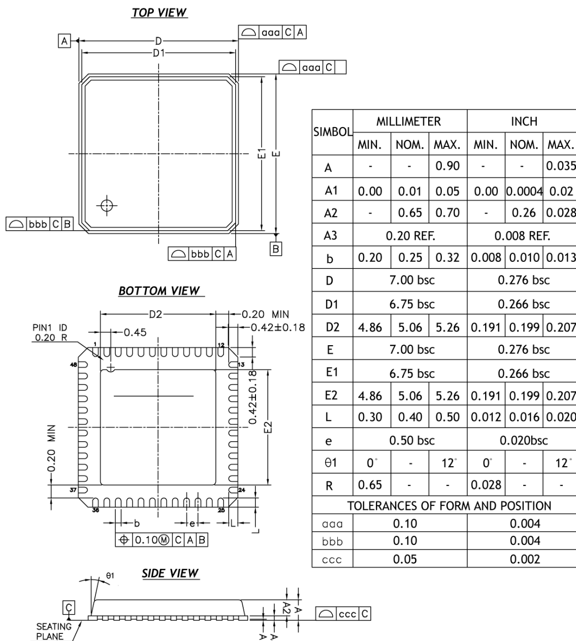
图 27 封装概述
