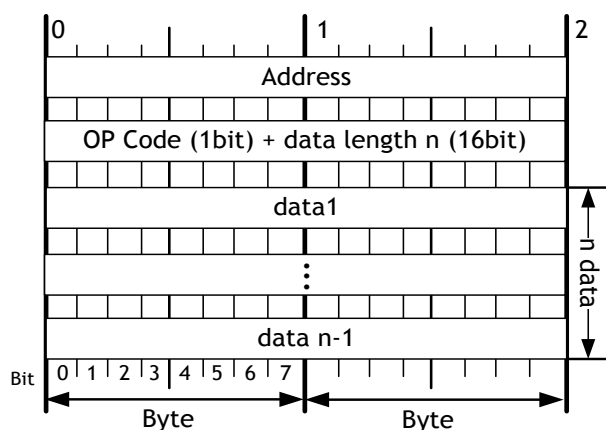
图 19 W5200 SPI帧格式
