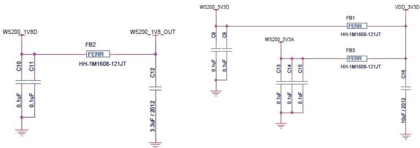
图 3 电源设计
