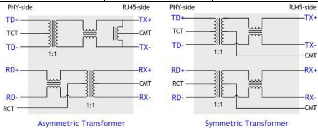
图 25 变压器特性
